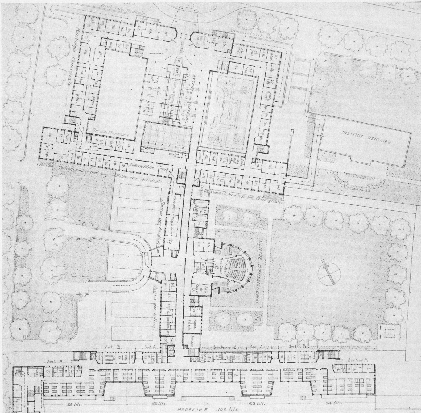
Fig. 18. Projet No. 10. Auteurs: A. ROSSIRE et F. DUC, architectes, Genève. Etage A, échelle 1:1000
