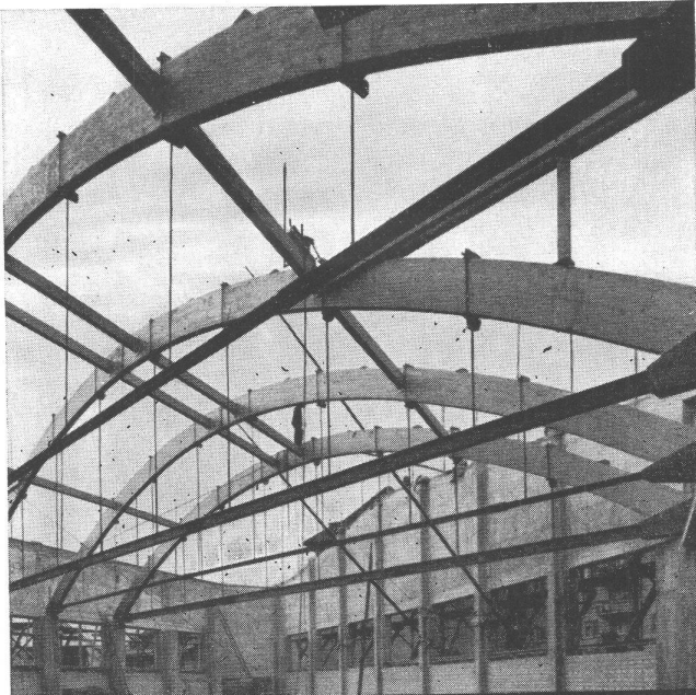
RINGDÜBEL + PATENT Knotenpunktverbindung für hölzerne Tragwerke
