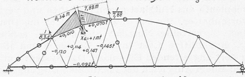
b. Momente u. Kräfte im Grundsystem für X_6 = +1 \text{ mt}
