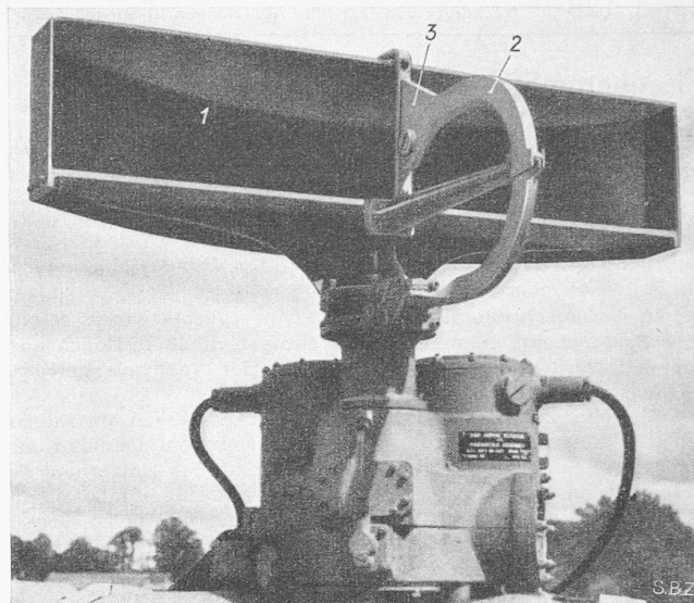
Bild 1. Antenne mit rotierendem «Kässchnitten»-Reflektor. 1 Reflektor, 2 Wellenleiter, 3 Trichter zum Einstrahlen der elektrischen Wellen in den Reflektor
