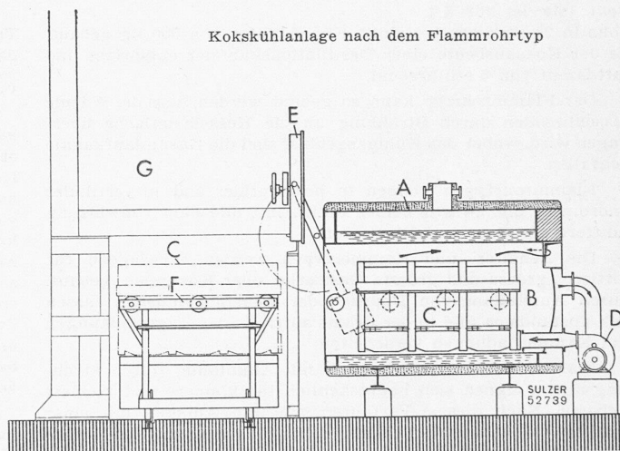
Bild 13. Schematischer Querschnitt. A Dampfkessel, B Kühlraum, C Kokskübel, D Gebläse, E Abschlussschalter, F Kübeltransportwagen, G Vertikalkammerofen
