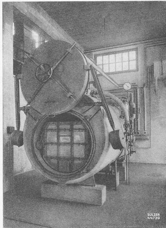
Bild 12. Bedienungsseite. Im Innern ist der Kokskübel sichtbar
