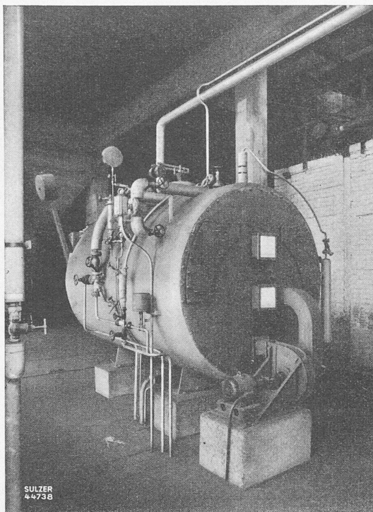
Bild 11. Gebläseseite, darüber Sicherheitsfenster
