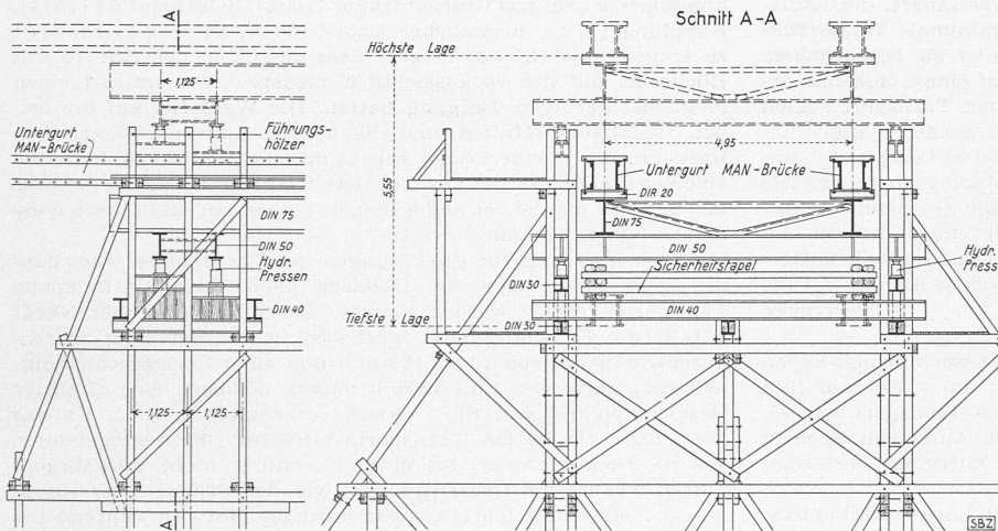
Bild 10. Hubvorrichtung auf dem Schiffsgestell, Masstab 1:150
