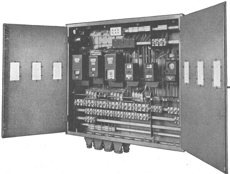
Vertellschrank mit abgehobener Isolierabdeckung
