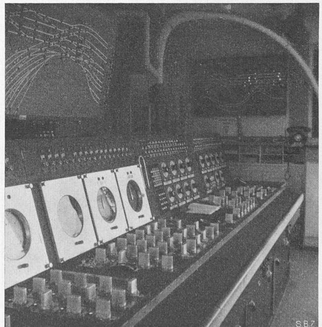
Bild 9. Stellwerk im Bahnhof Bern-PB, das modernste im Netz der SBB. Unten Vierreihen-Schalterwerk, darüber Gleistafel, hinten Fahrtafel auf der Westseite
