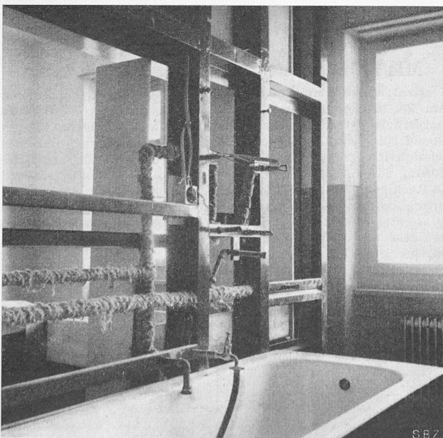
Bild 3. Isolierung der Leitungen
