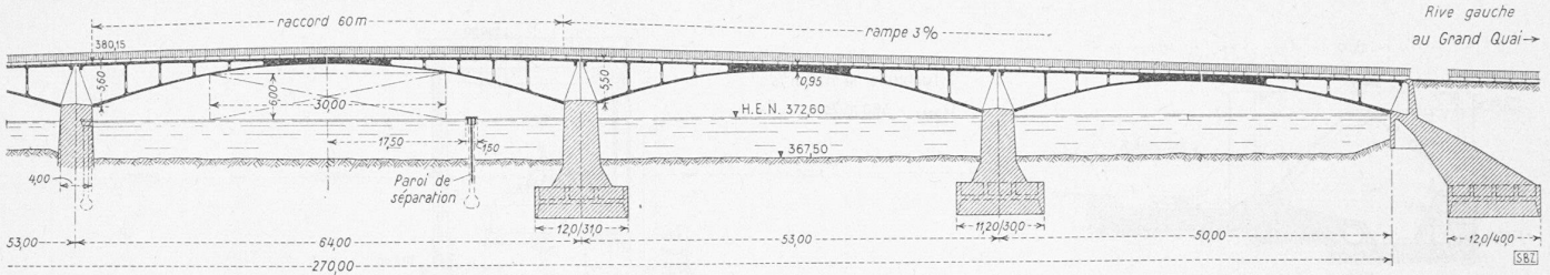
Bild 10. Neue Mont-Blanc-Brücke; Längsschnitt der linksufrigen Hälfte 1:1000. Leichte Eisenbeton-Gewölbe mit kastenförmigem Querschnitt. Schifffahrt-Profil der Mittelöffnung 30 × 6 m
