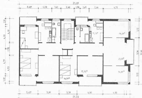
3 OBERGESCHOSS
