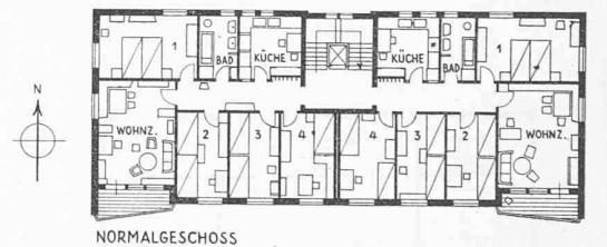
NORMALGESCHOSS
