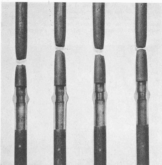
Bild 9. ZerreiBproben an Rohrausschnitten mit Schweißungen
