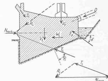
Bild 16. Zeichnerische Ermittlung der Riegelkraft N_{vorh} (linkes Widerlager)
