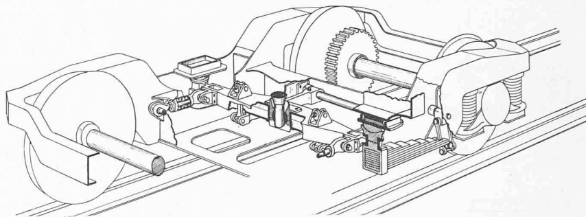
Bild 10. Triebdrehgestell der F 0 4/4-Triebwagen, geliefert 1938/39 von der SLM ursprünglich an die SBB
