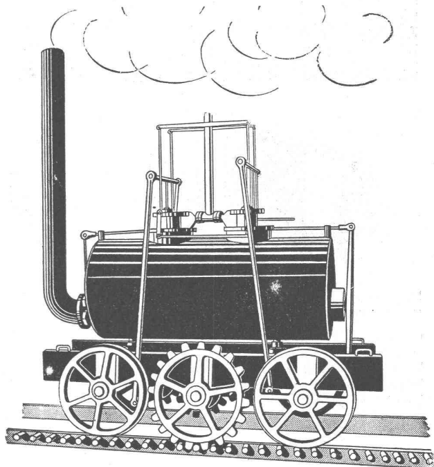
Lokomotive von Blenkinsope 1812, lief 5 km/St.
