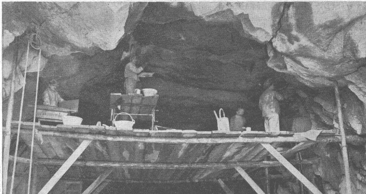
Dichtung von Infiltrationen in Granitquaderwerk mit Barra
