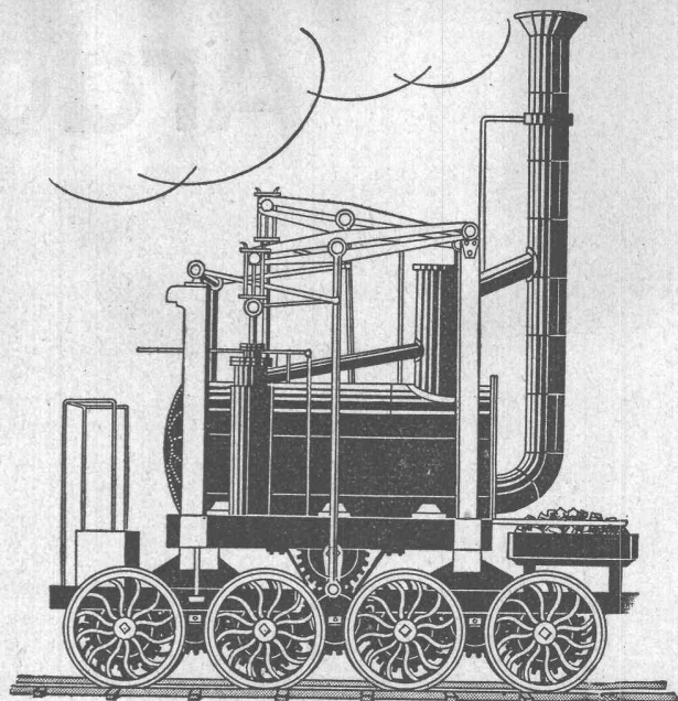
1815: Hedley's 2. Lokomotive besaß 4 Triebachsen mit Zahnradübertragung
