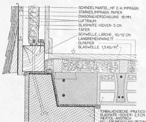
Bild 23. Vertikalschnitt: Aussenwand Anschluss an das massive Kellergeschoss
