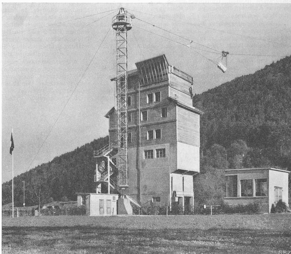
Bild 8. Aufbereitungsanlage Lüttau von Norden, rechts Windenhaus, vorn Transformatorenstation
