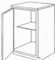
Bild 32. Unterschränk HSB-BORO mit einem festen Tablar. Masse: Breite 45, 60 cm, Höhe 80 oder 90 cm, Tiefe 57 cm
