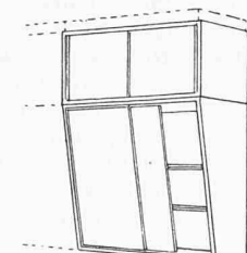
Bild 26. Oberschrank-Einheit der neuen HSB-Standard- Küche, Bild 5. Masse: 100 × 120 × 22 bis 39 cm
