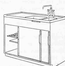
Bild 28. Spültisch-Einheit HSB-BORO. Masse: 120 × 57 cm, Höhe 80 und 90 cm
