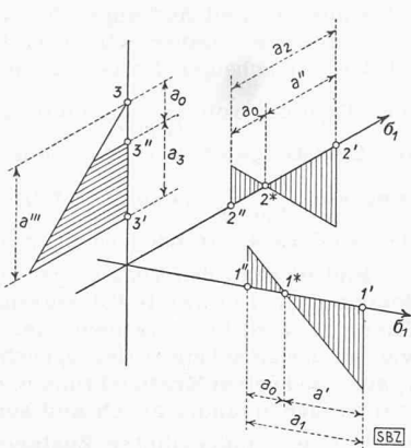
Bild 9. Axonometrische Darstellung der Gitterspannungen und Dehnungen an der zweiten Fließgrenze des zweiachsigen Belastungszustandes \sigma_1 = \sigma_2, \sigma_3 = 0
