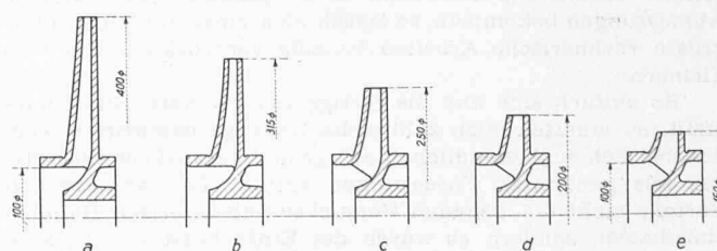
Bild 9. Genormte Kreisel-Pumpen-Laufräder
