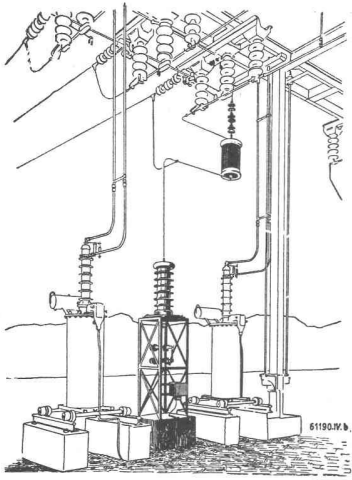
HF-Telephonieschrank für ein Kraftwerk u. zugehörige Ausenanlage mit dem Kopplungskondensator (Mitte) und der Hochfrequenzsperre (rechts oben).
