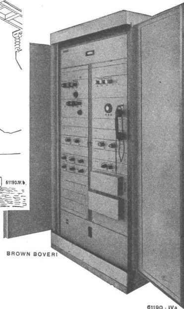
HF-Telephonieschrank für ein Kraftwerk u. zugehörige Ausenanlage mit dem Kopplungskondensator (Mitte) und der Hochfrequenzsperre (rechts oben).
