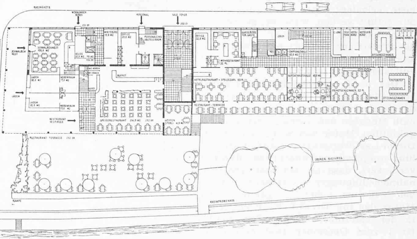
Grundrisse Erdgeschoss und erstes Obergeschoss, 1:800
