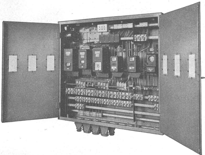
Verteiltschrank mit abgehobener Isolierabdeckung
