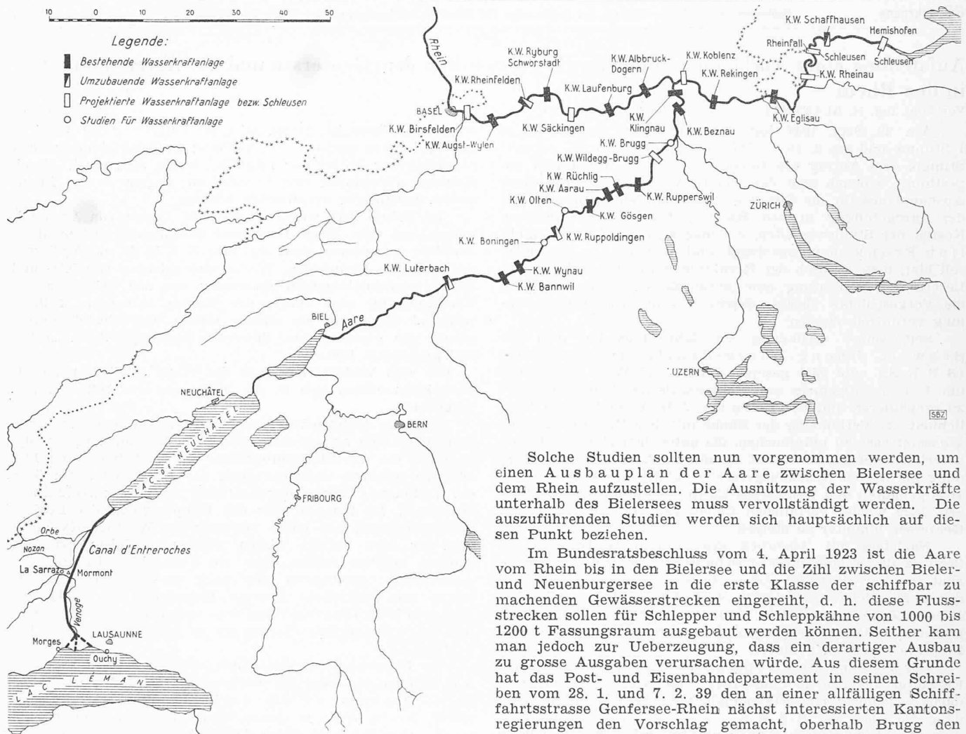
Bild 1. Der transhelvetische Kanal und die Wasserstrasse Basel-Bodensee, Projektskizze 1:1100000
