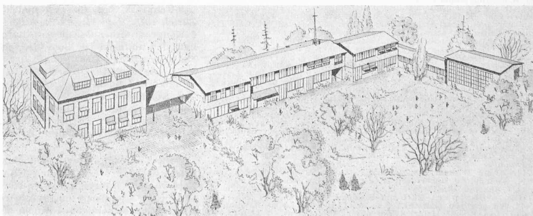
3. Preis. Erdgeschoss 1:600 (Abwartwohnung über Handfertigkeit). Unten Isometrie aus Süden
