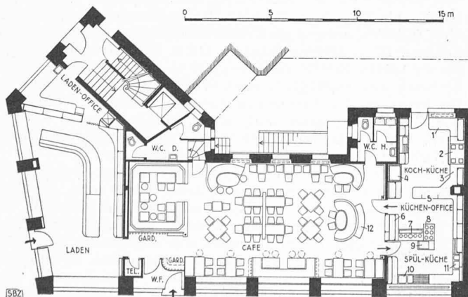
Bild 1. Grundriss 1:300. Legende: 1 Rüsten, 2 Kochen (bestehend Gasher), 3 Anrichten, 4 Kühlschrank, 5 Wärmeschrank, 6 Getränke, 7 Kaffeemaschine, 8 Glace, 9 Reg.-Kasse, 10 Gläserspüle, 11 Geschirrspüle, 12 Besteck. — Laden siehe Seite 126
