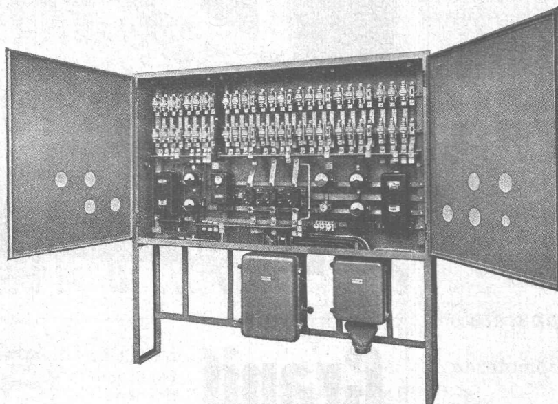
Vertellschrank mit abgehobener Isolierabdeckung
