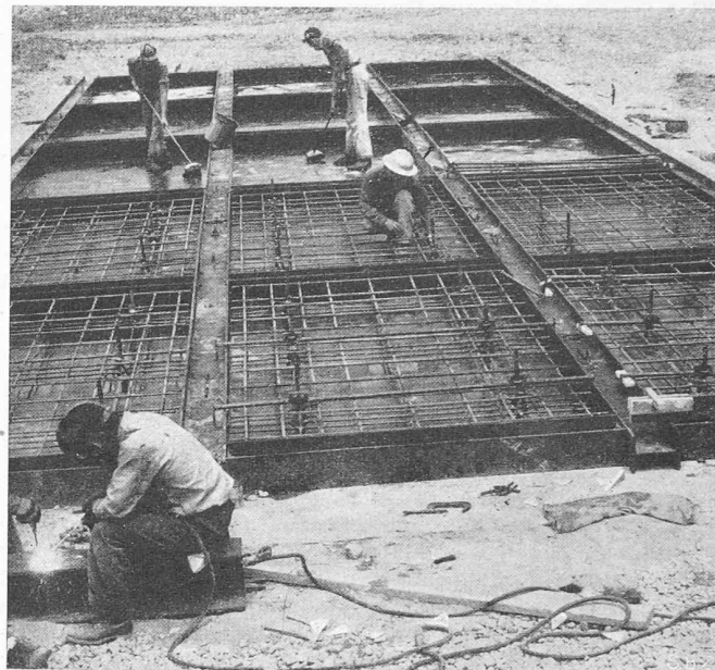
Bild 1. Herstellung vorgegossener, armerierter Betonplatten für die Bekleidung der wasserseitigen Oberfläche
