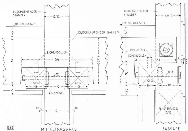
Bild 1. Anschluss der Balken an die durchgehenden Ständer; Detail 1:10
