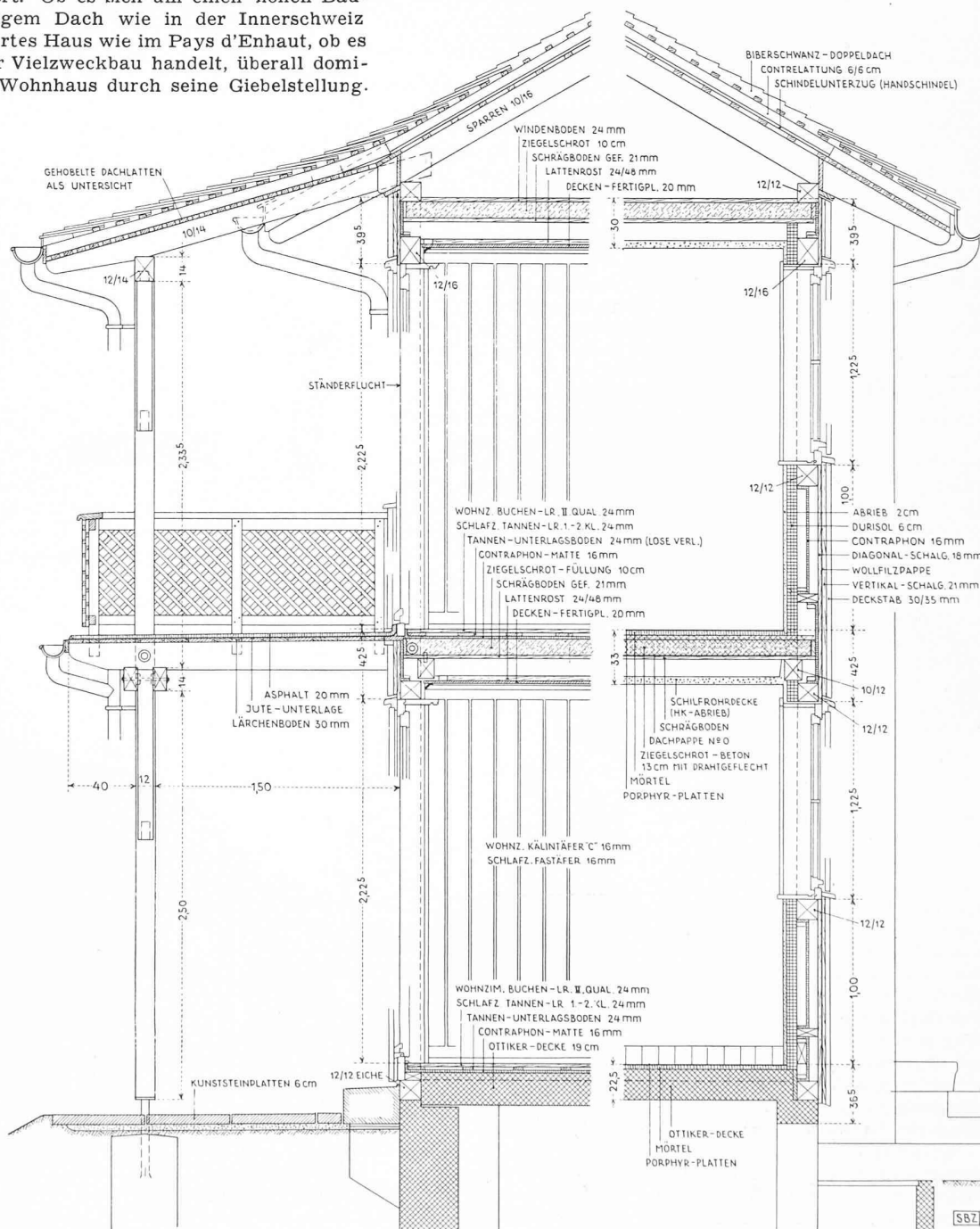
Bild 2. Siedlung im «Schachen» in Winterthur; Arch. FRANZ SCHEIBLER. Querschnitt des Zweifamilien-Hauses, Masstab 1:40. Text siehe Seite 349
