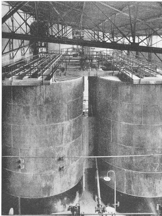
Bild 4. Rohschlambottiche
