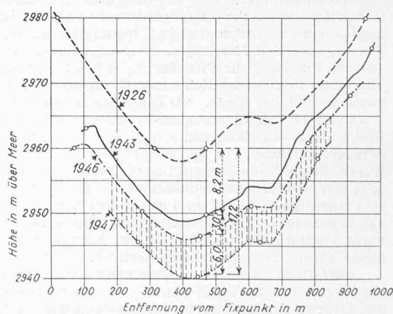
Bild 9. Höhenänderungen der Firnoberfläche in Profil Firn (Fixpunkt linkes Ufer 2998 m, vgl. Bild 1)
