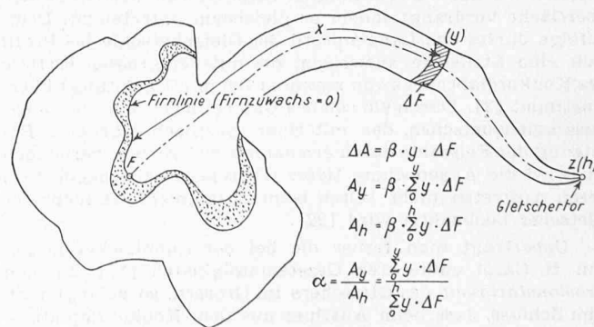
Bild 18. Näherungsweise Bestimmung der verhältnismässigen Zunahme \alpha des jährlichen Wasserabflusses infolge Ablation zwischen Firnlinie und Gletscherort. \beta = Proportionalitätsfaktor, y = Höhendifferenz zwischen Firnlinie und Element \Delta F
