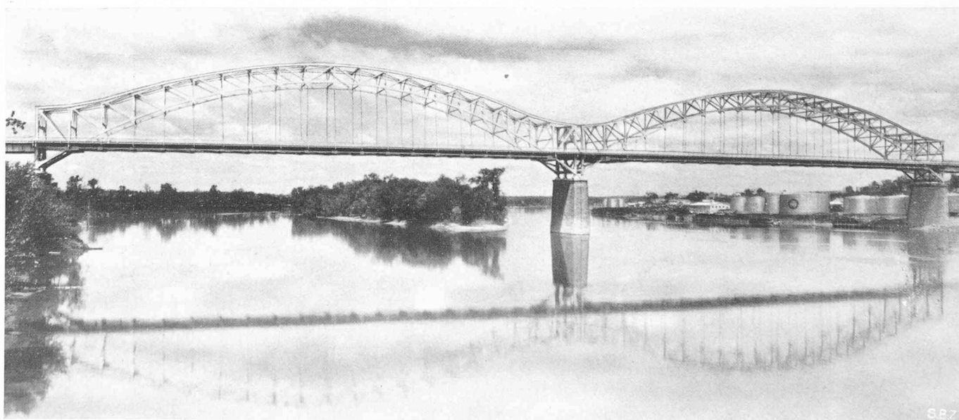
Bild 23. Fachwerkbogen mit Zugband über den Connecticut River bei Middletown
