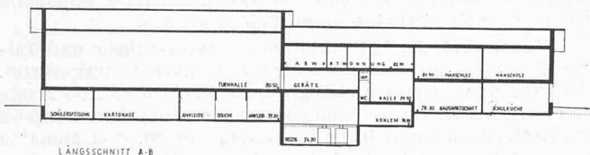
LÄNGSSCHNITT A-B
