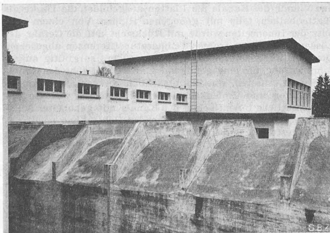
Bild 31. Verbindungssteg, darunter grosser Windkanal; hinten grosse Messhalle, ganz rechts Trudelturm
