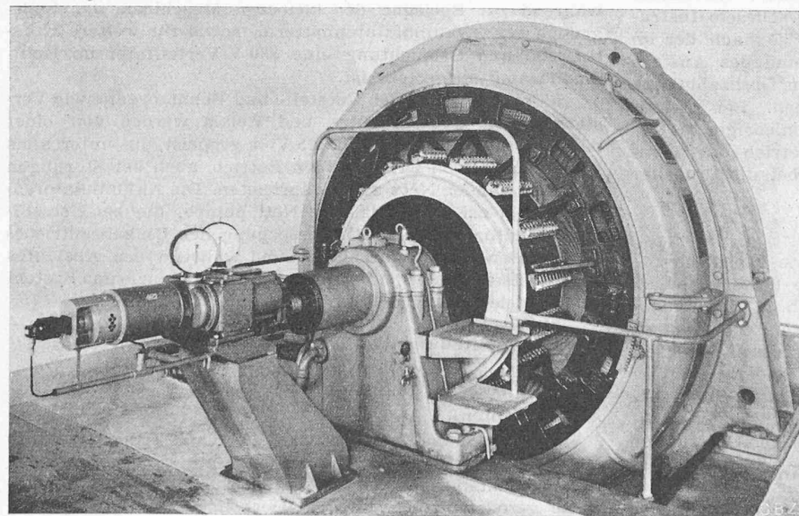
Bild 25. Betriebsmotor des grossen Gebläses mit angebautes Reguliergetriebe, Kontrolltachometern und Steuerfrequenzgenerator
