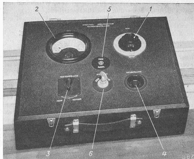
Bild 19. Tragbarer Steuerkasten für den Gebläseantrieb. 1 Drehzahl-Einsteller, 2 Stellungsferrnanzeiger der Feineinstellung, 3 Feineinsteller «Mehr — 0 — Weniger», 4 Notknopf, 5 Umschalter «Hand» — «automatisch», 6 Sicherheitsschlüssel
