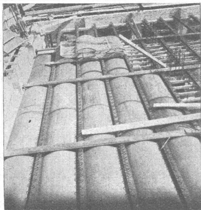
Deckenschalung für Fabrikdecke von oben
