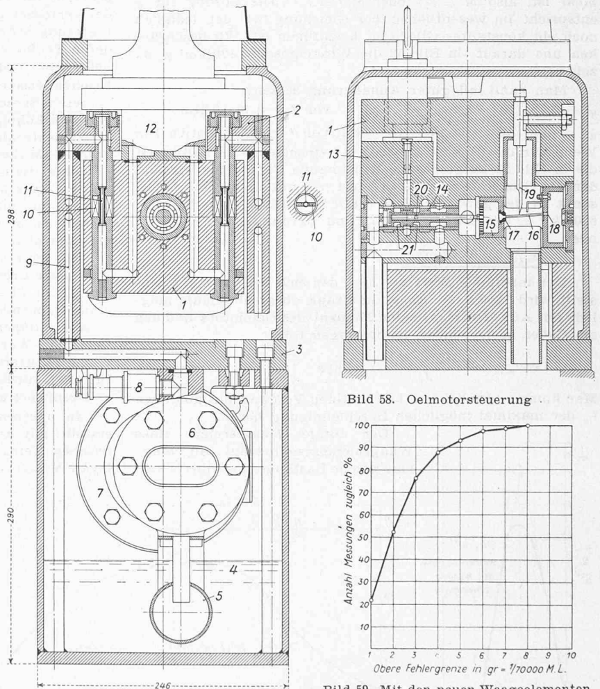
Bild 57. Neuere Ausführung der Waageelemente
