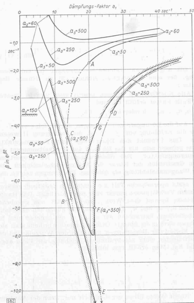
Bild 48 (links). \beta -Kurven in Abhängigkeit der Dämpfung a_1 der Federung a_2 und des Steuerfaktors a_3
