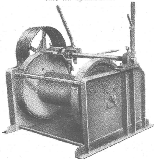
Seilwinden KS für Zugkraft von 1,5 und 2,5 Tonnen
