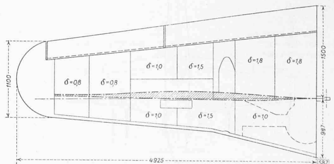
Bild 6. Flügelgrundriss mit Streubereich der elastischen Axen
