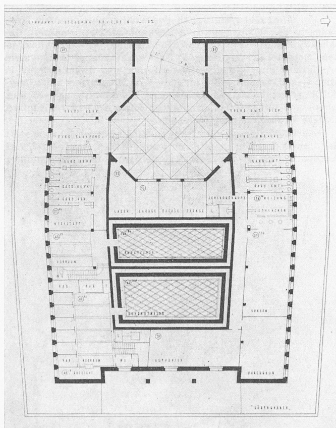
Untergeschoss 1:600
