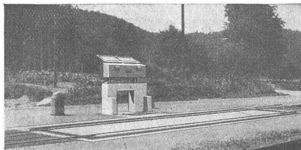
Brückenwaage für Geleise- u. Strassenfahrzeuge, Wiegefähigkeit 40 t. Normaltyp SBB mit armerter Betonbrücke in Rippenkonstruktion Bauart Giroud Länge 8,4 m, befahrbar mit allen Verkehrslasten
