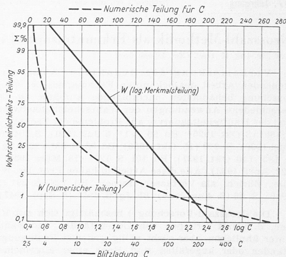
Bild 2. Verteilung der Ladung von Blitzschlägen (nach McEachron ) in verschiedener Darstellung
