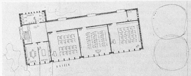
2. Preis (2200 Fr.) HERMANN BAUR, Arch., Basel. Südansicht, Erdgeschoss und Obergeschoss 1:600, unten Perspektive aus Osten. Text siehe Seite 283
