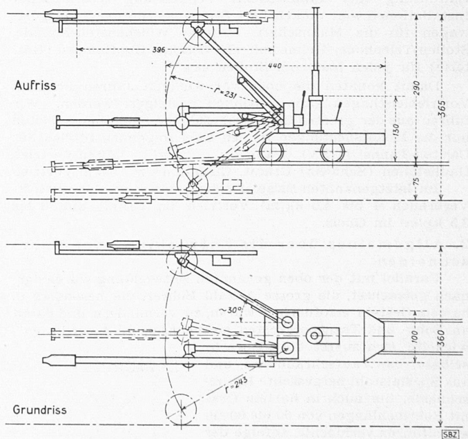
Bild 3. Bohrswagen SULLIVAN-JOY mit zwei Auslegern und Lafetten von 4 m Länge (die Lafetten werden auch in Längen von 2,20, 2,80 u. 3,40 m geliefert) Massstab 1:100
