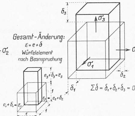
Bild 2. Gesamte Änderung des Körperelementes als Überlagerung der elastischen Formänderung und der plastischen Verformung
