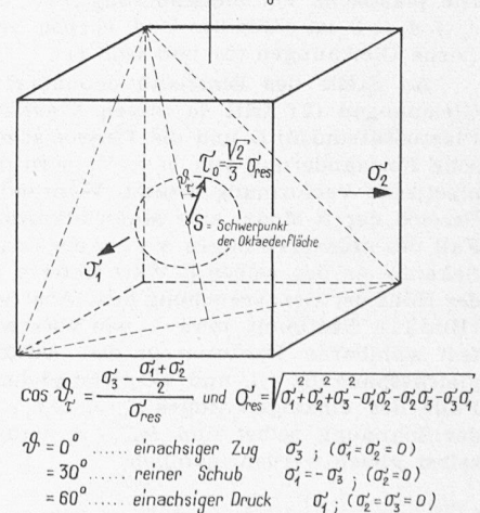
Bild 7. Orientierung der Schubspannung \tau_0 in der Oktaederebene
