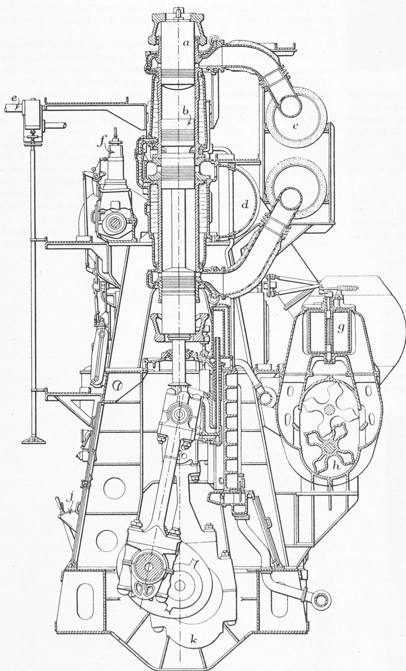
Bild 1. Querschnitt durch einen doppelwirkenden Zweitakt-Schiffs-Dieselmotor, Bauart Harland & Wolff, von 1000 PS Zylinderleistung. Masstab 1:60
