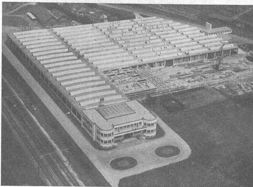
Traktoren- und Motorenwerke H. Hürlimann, Wil - Erweiterung 1946—1949, Flachbedachung 10 000 m 2 Bauleitung: F. Vogt, Architekt, Wil — Bauunternehmung: Ed. Züblin & Cie. A.-G., Zürich
