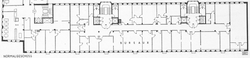
Bild 18. Normalgeschoss, Masstab 1 : 600
